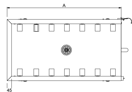
Boven aanzicht
